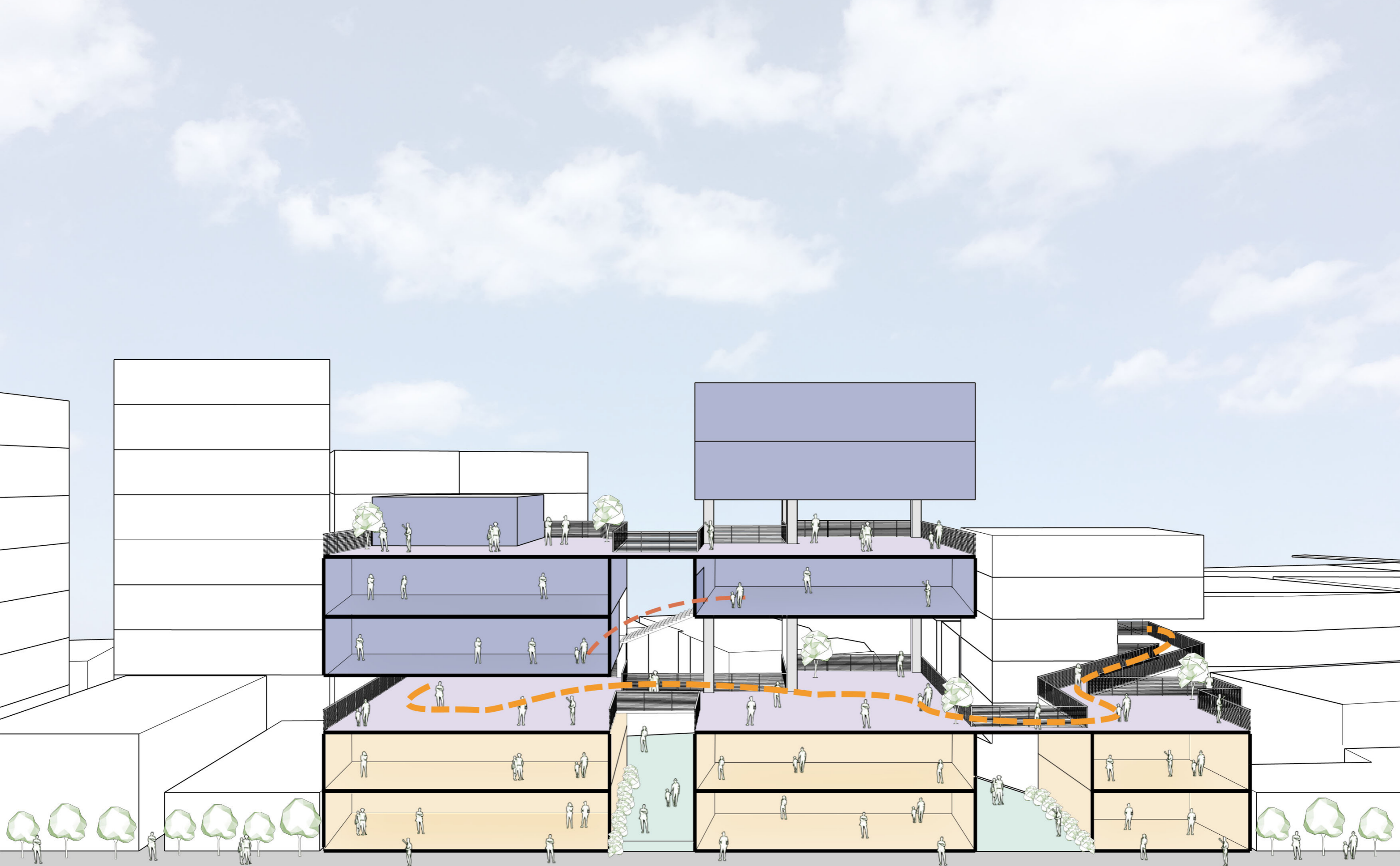
Section through vertical alleys 수직적 골목 단면
